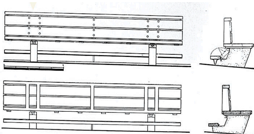
Acima : projeto dos bancos da nossa igreja
